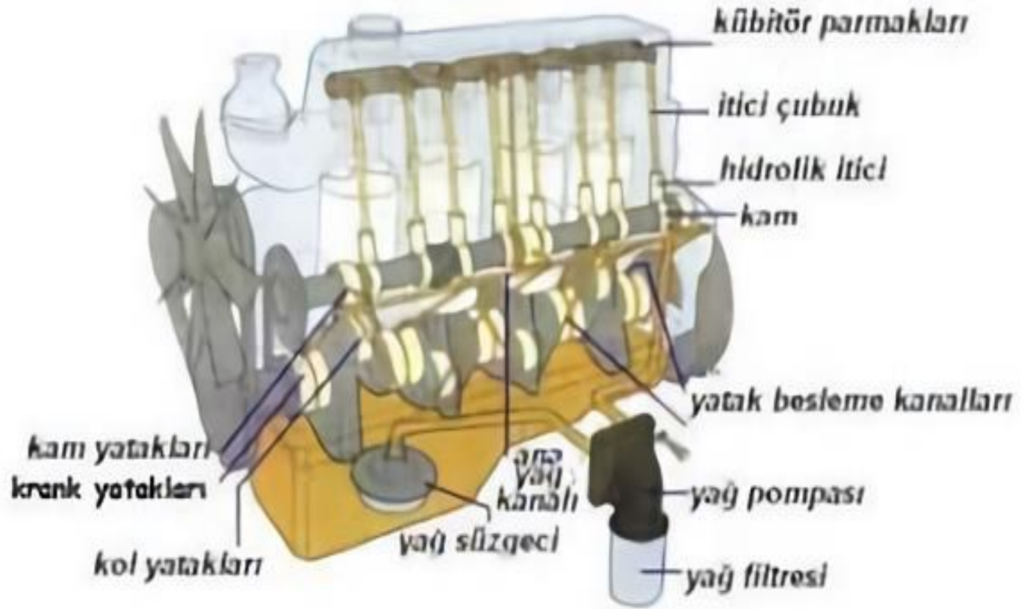
Motorum Yağlama Sistemi ve Parçaları.
